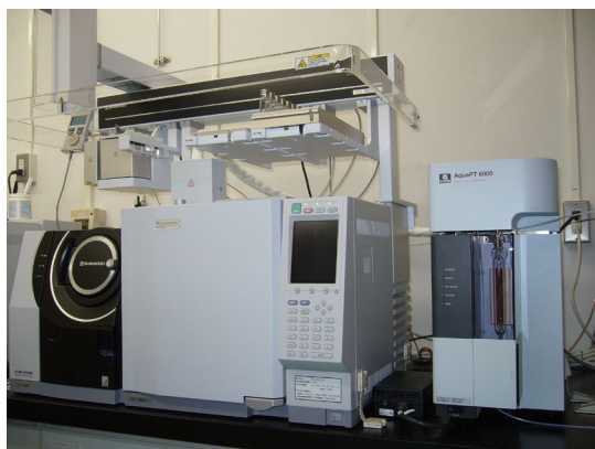
かび臭物質の測定に使用するガスクロマトグラフー質量分析装置
